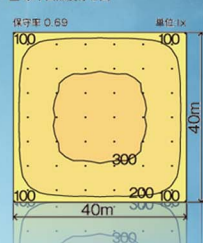
■ 水平面照度分布図
