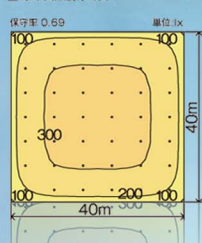
■ 水平面照度分布図
